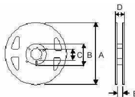
Reel Dimensions
