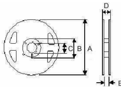
Reel Dimensions
