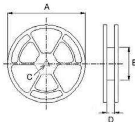
Reel Dimensions
